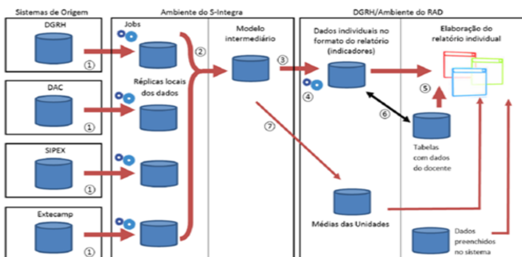
Esquema 1. Esquema do modelo de geração dos dados do RAD
